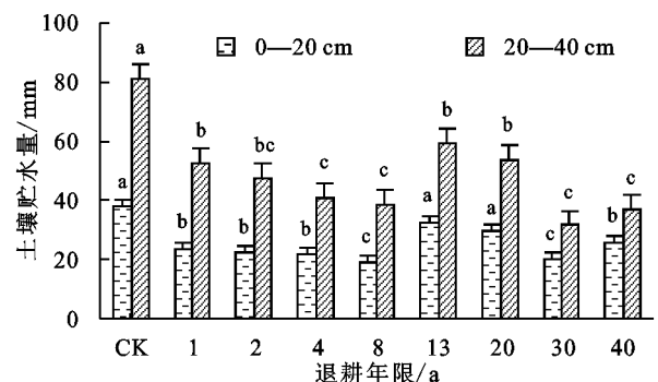
图 1 不同年限退耕地土壤水分特征
