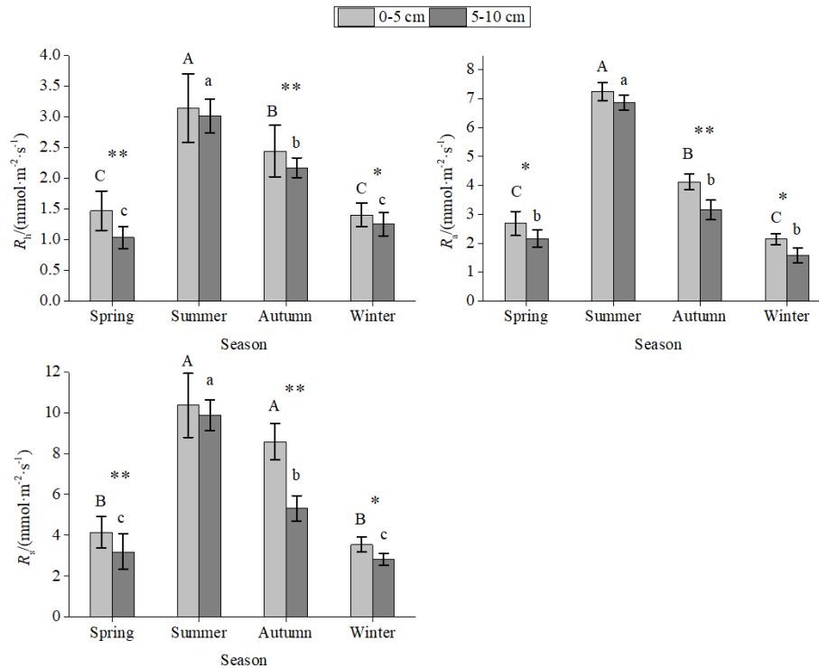
图2 西双版纳热带季节雨林土壤总呼吸 ( R_s )、自养呼吸 ( R_a ) 及异养呼吸 ( R_h )
