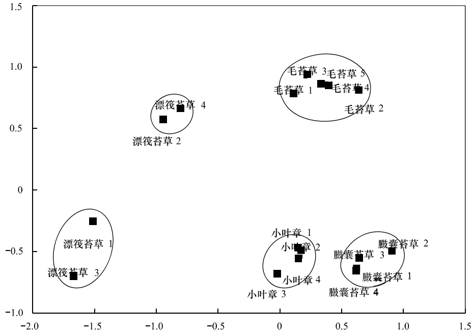
图 2 不同类型湿地螺类集合的非度量多维标度序图
