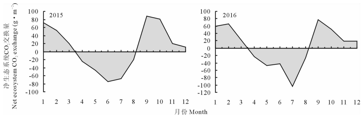
图3 2015和2016年生态系统净CO 2 交换量(NEE)月变化
