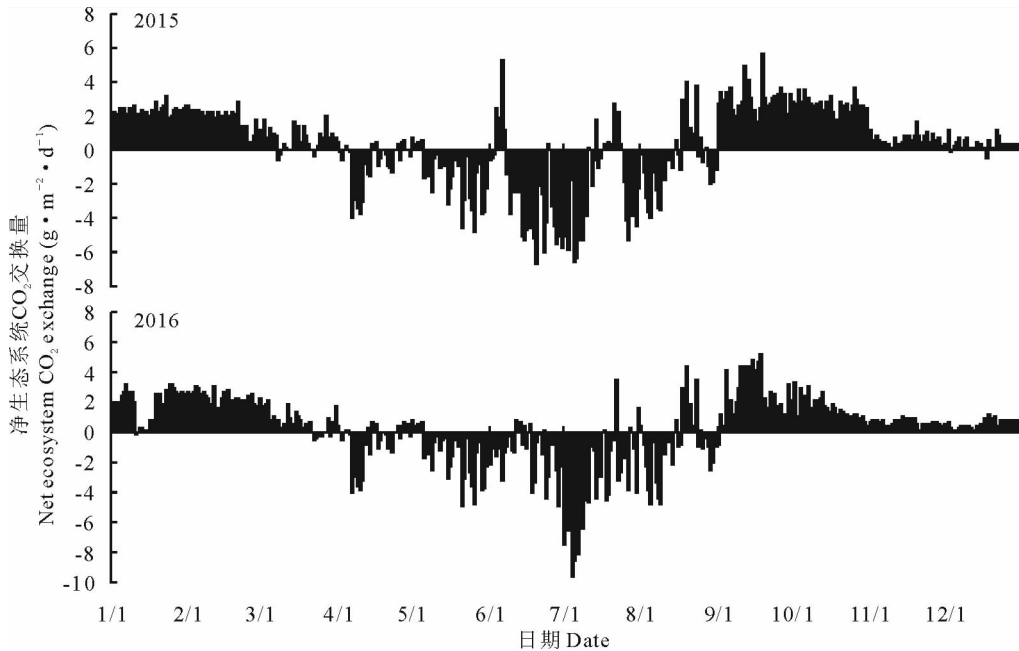
图 2 2015 和 2016 年生态系统净 \text{CO}_2 交换量(NEE)逐日变化 Fig. 2 Variation of diurnal net ecosystem \text{CO}_2 exchange (NEE) during 2015 and 2016
